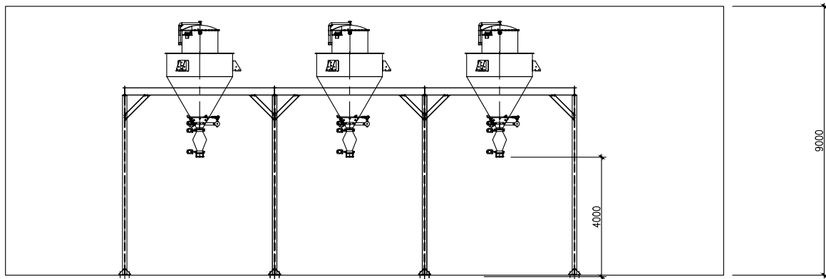
主视图
