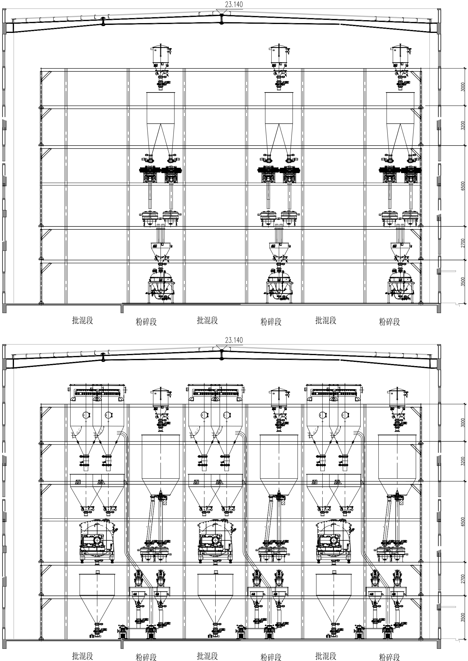
主视图
